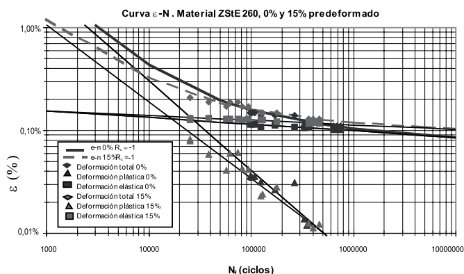
Figura 4. Curvas \epsilon -N de Material ZStE 260.
