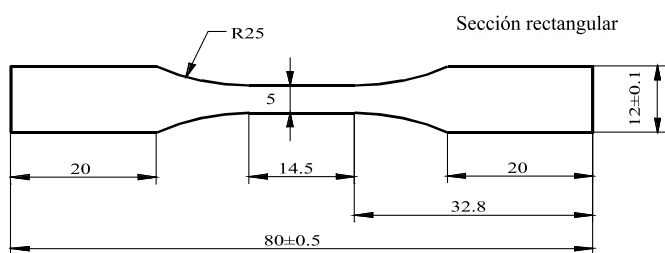
Figura 1. Probeta de ensayo. Dimensiones en mm.
